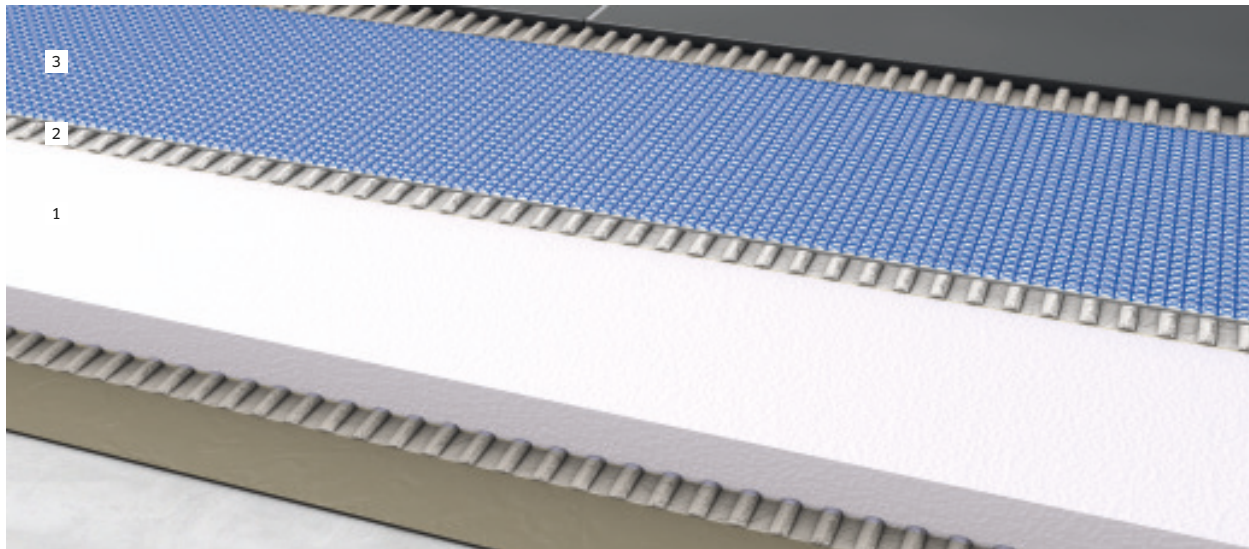
SYSTEMBESTANDTEILE 1 BLANKE PERMATFLOOR Dämmung 2 BLANKE GLUEMAX 3 BLANKE PERMAT inkl. Randdämmstreifen
