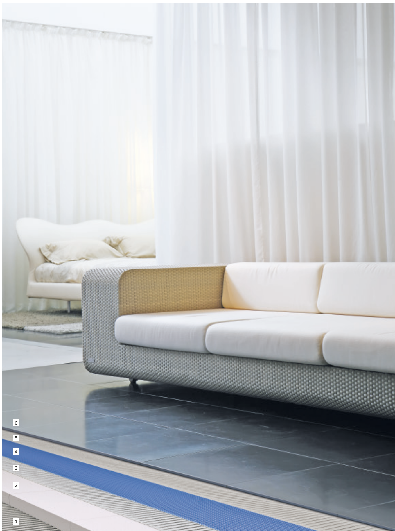
1 Flexklebermörtel 2 BLANKE PERMATFLOOR Dämmung 3 BLANKE GLUEMAX 4 BLANKE PERMAT 5 Flexklebermörtel 6 Oberbelag
